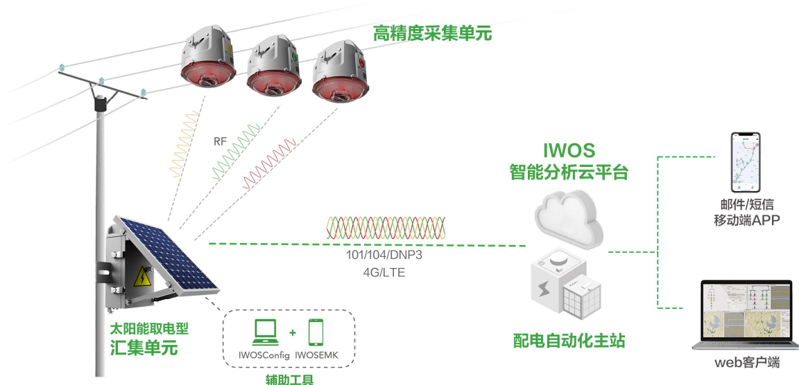
智能化配电网线路状态监测系统
