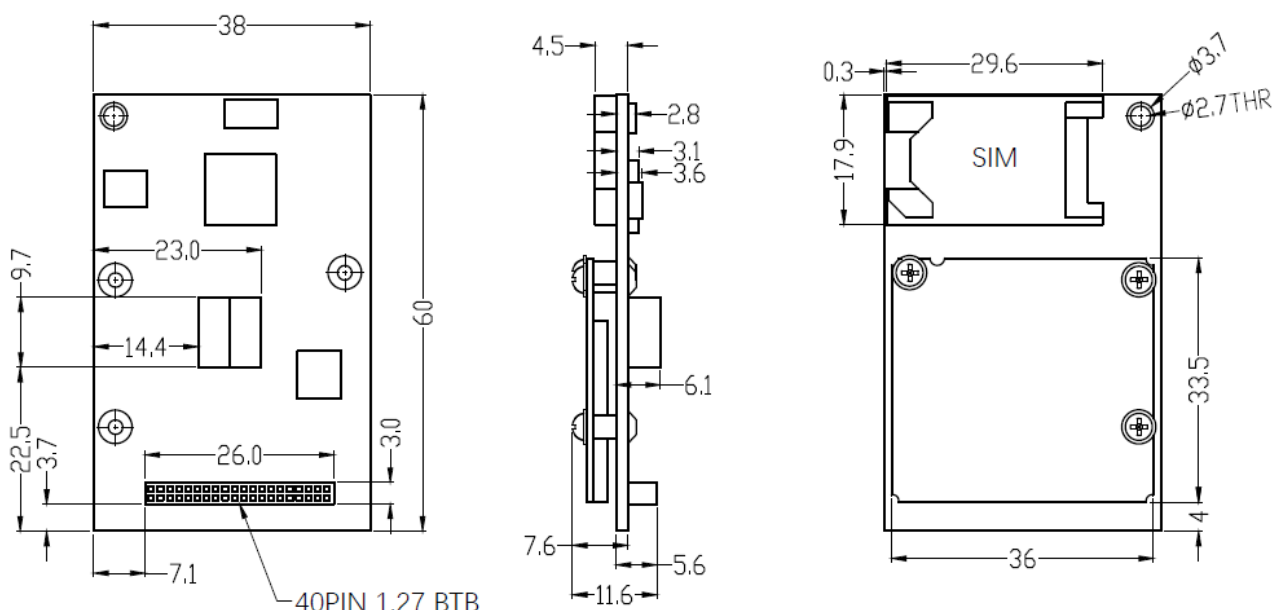
InDTU323G 的尺寸
