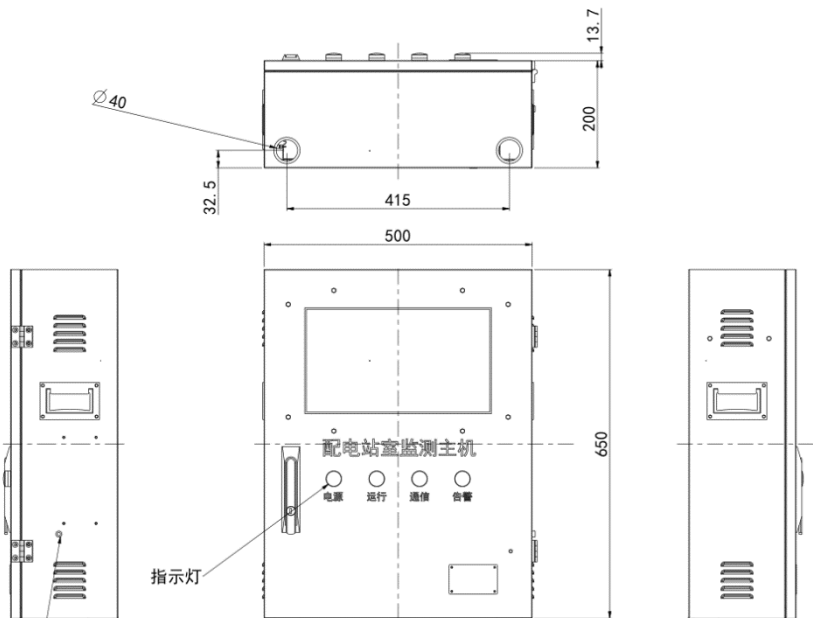
尺寸（长*宽*高）：500*200*650mm
