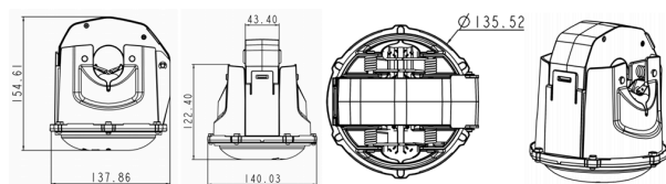
尺寸（长×宽×高）：138mm×140mm×155mm
