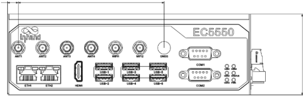
接口图
