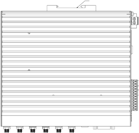
侧视图
