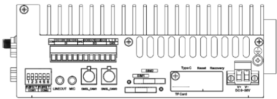
侧视图
