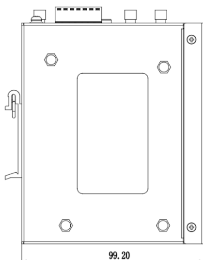
正视图
