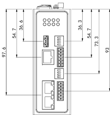
接口图
