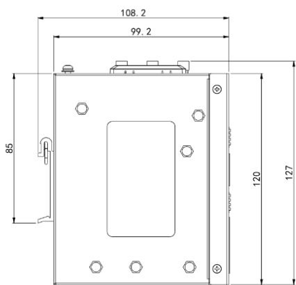
正视图
