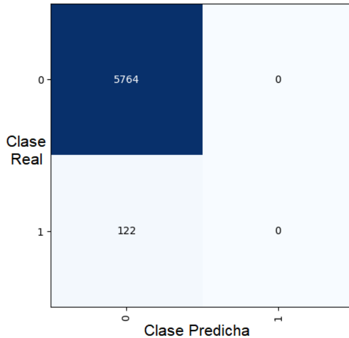
Figura 5: Visualización de la matriz de confusión sobre el conjunto completo (concretamente la del modelo Deit ).
