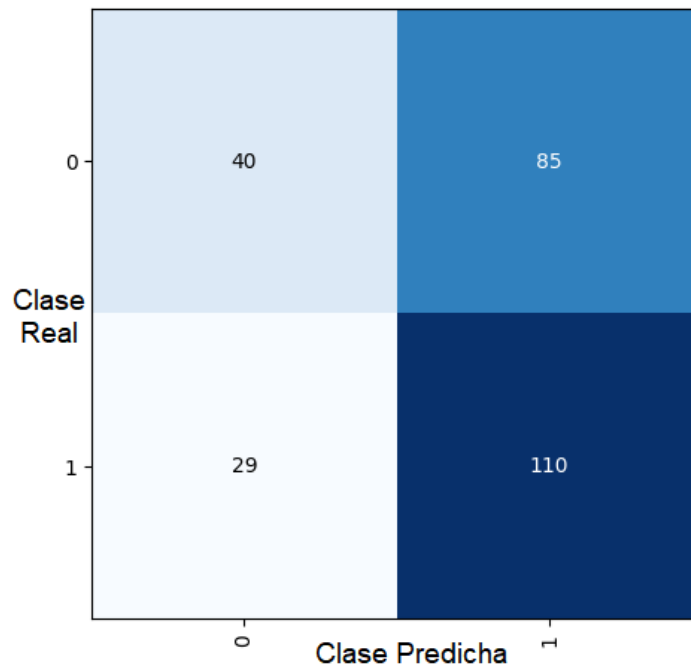
Figura 6: Visualización de la matriz de confusión sobre el conjunto balanceado (concretamente la del modelo ResNet ).
