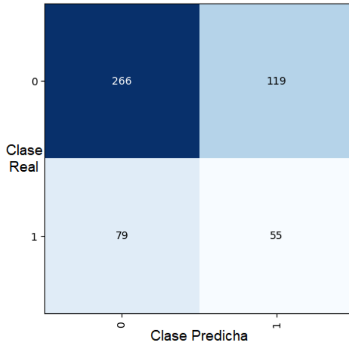
Figura 9: Visualización de la matriz de confusión sobre el conjunto balanceado por pacientes (concretamente la del modelo ConvNext ).
