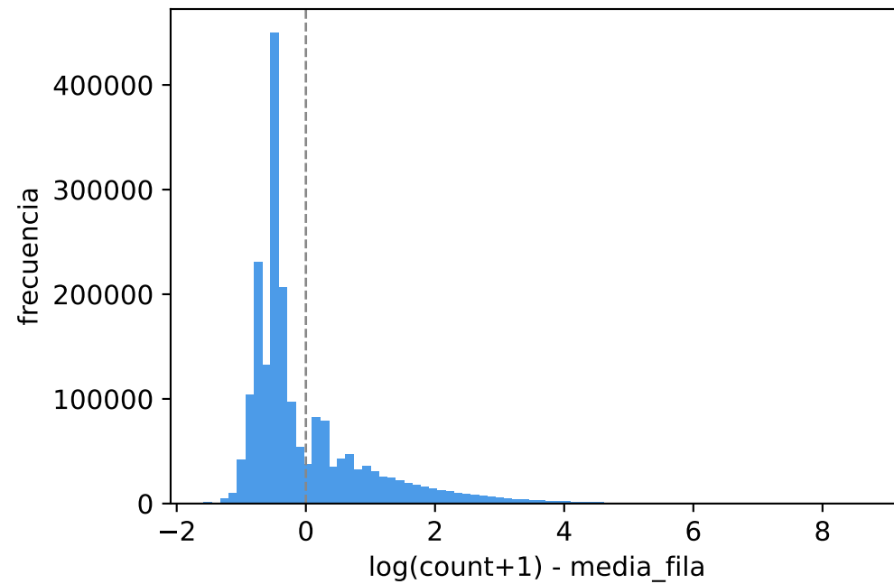
4. Tras CLR (centrado por fila) skew=2.02 mean=-0.00 sd=0.98
