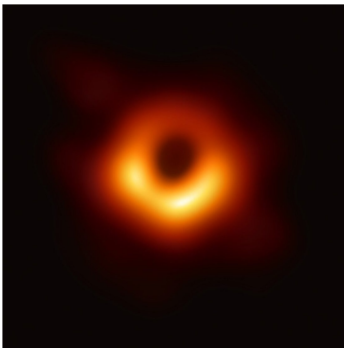
La sombra de M87*, la primera imagen de un agujero negro (Event Horizon Telescope, 2019)
