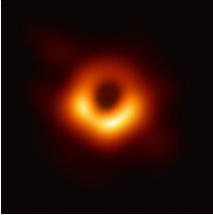
Primera imagen directa del horizonte de sucesos de un agujero negro, captada por el Event Horizon Telescope en 2019. El anillo brillante es gas caliente orbitando el horizonte; la sombra oscura central es el propio horizonte. La imagen confirma las predicciones de la relatividad general con una precisión sin precedentes. Crédito: EHT Collaboration.
