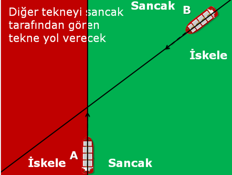
Şekil 2.4 — Aykırı Yaklaşma (MEB Denizcilik/COLREG modülü)
