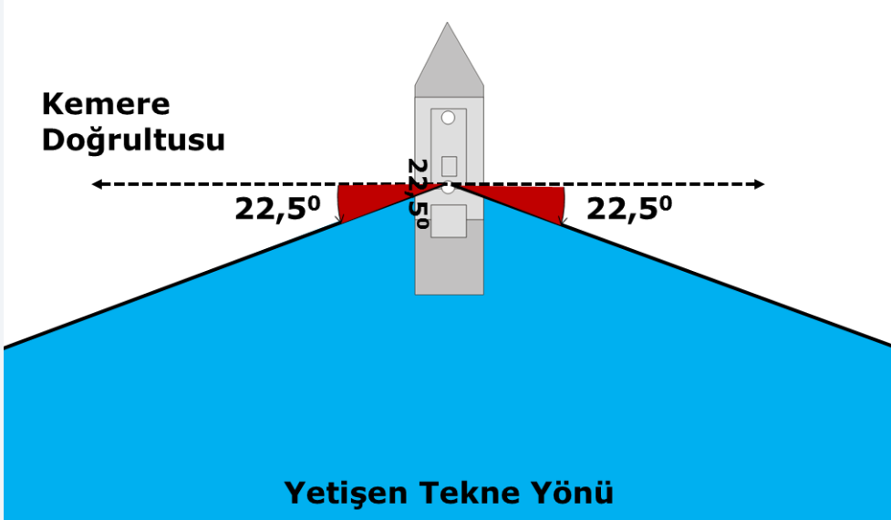
Şekil 2.2 — Yetişen Tekne Yönü (MEB Denizcilik/COLREG modülü)
