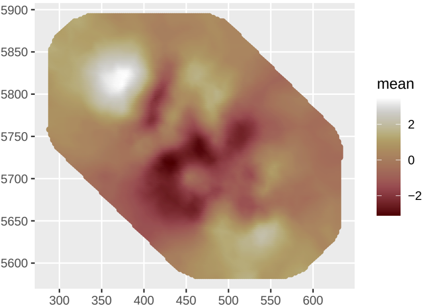
Posterior mean
