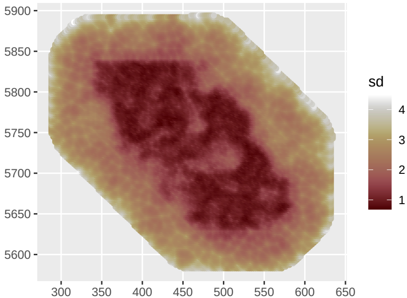
Posterior sd
