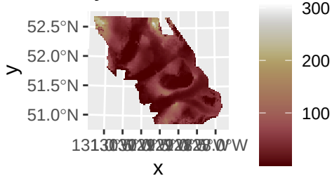
Posterior mean for catch probability
