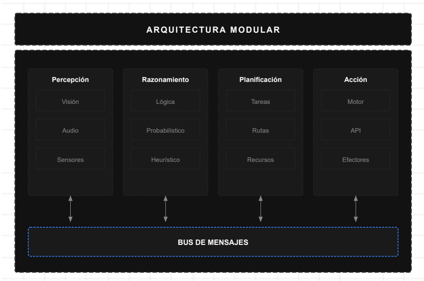
Figura 9: Arquitectura Modular
