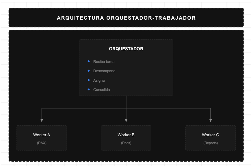
Figura 11: Arquitectura Orquestador-Trabajador
