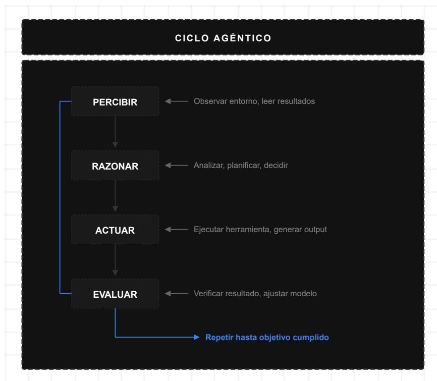
Figura 3: Ciclo Agéntico
