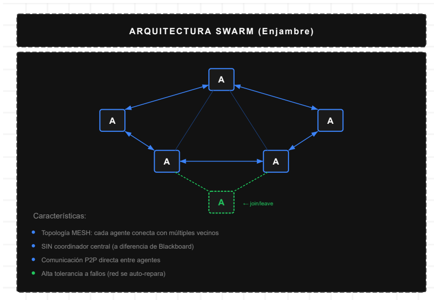
Figura 7: Arquitectura Swarm
