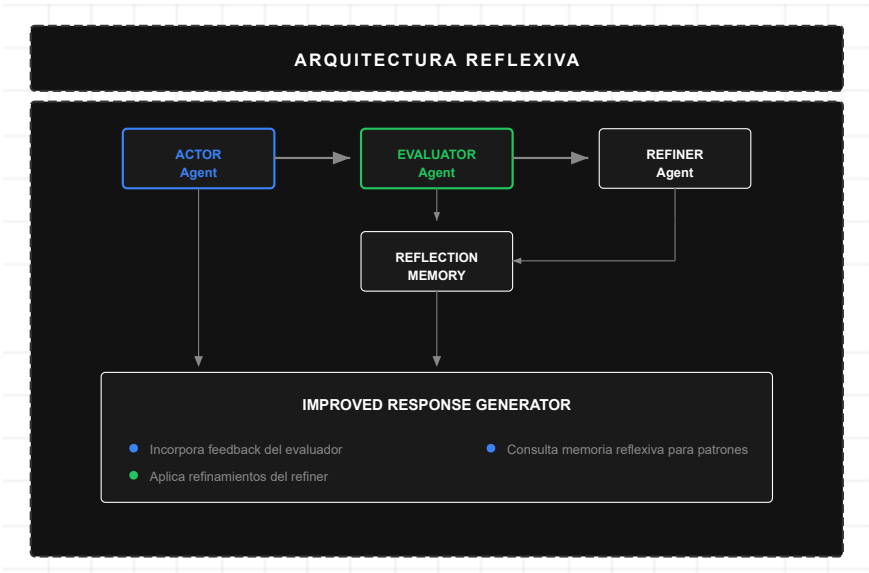
Figura 16: Arquitectura Reflexiva
