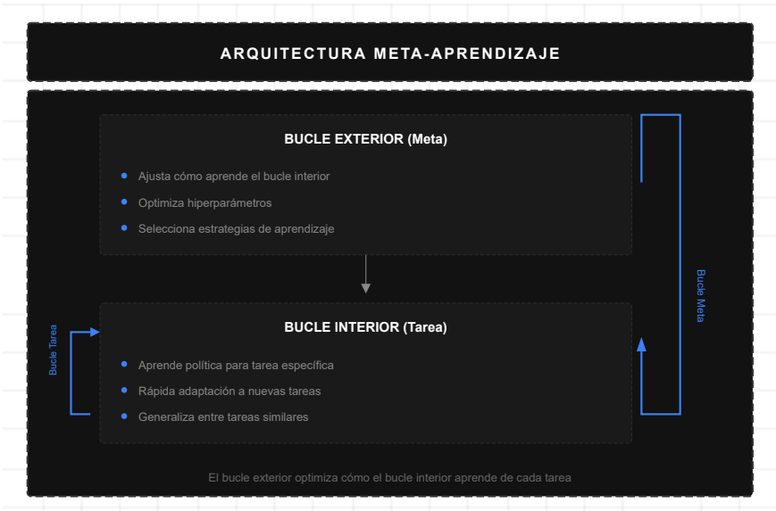
Figura 8: Meta-Aprendizaje
