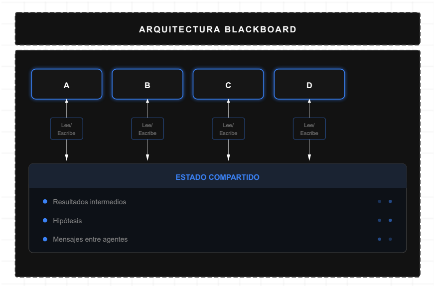
Figura 13: Arquitectura Blackboard
