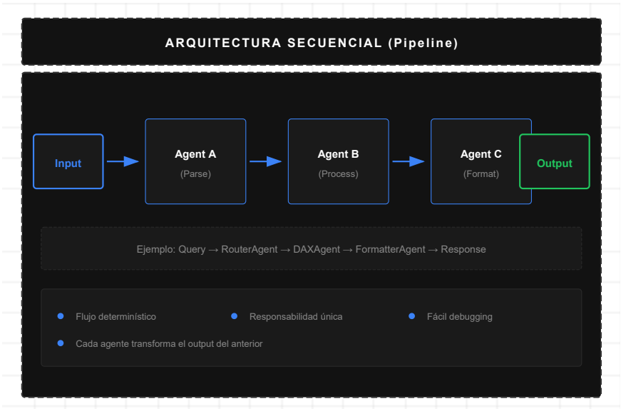
Figura 14: Arquitectura Secuencial
