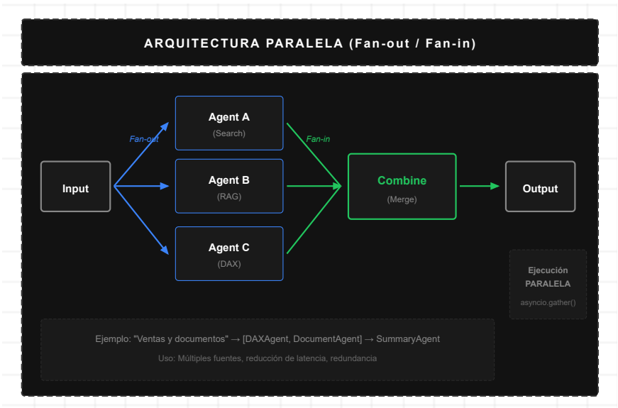
Figura 15: Arquitectura Paralela
