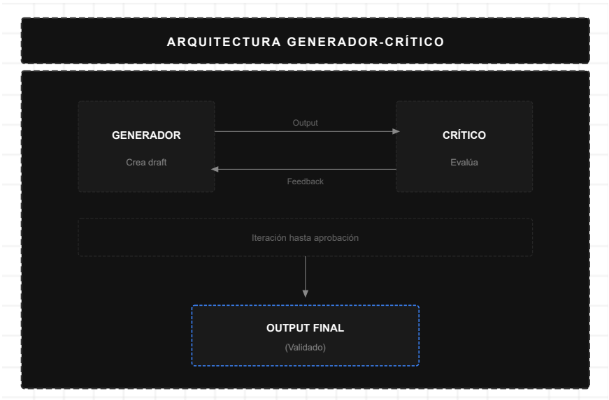
Figura 12: Arquitectura Generador-Crítico
