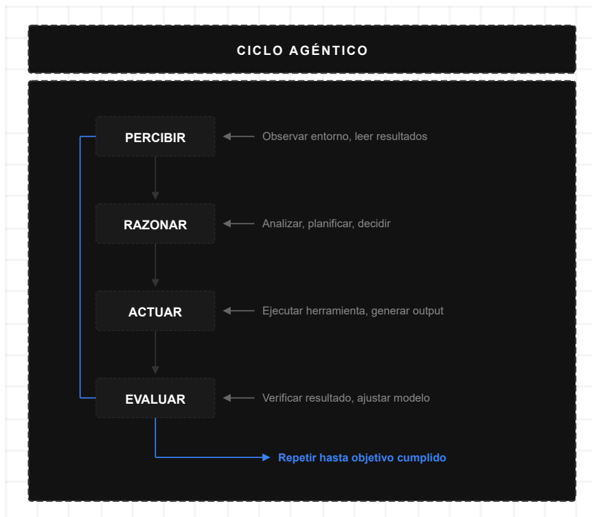
Figura 3: Ciclo Agéntico
