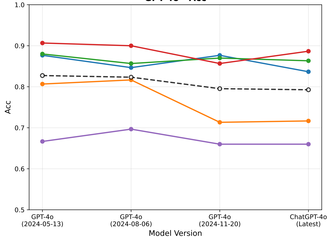
GPT-4o - Acc
