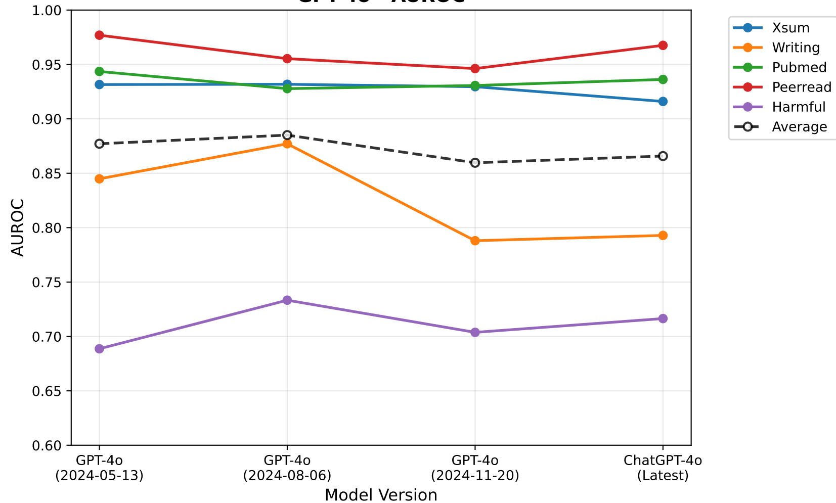
GPT-4o - AUROC
