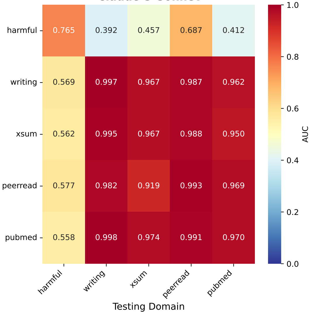
Claude-3-Sonnet
