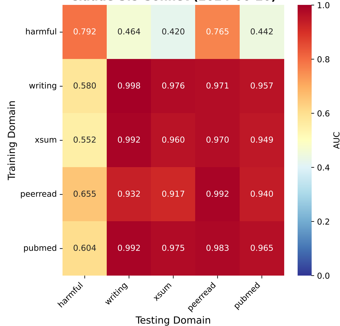
Claude-3.5-Sonnet (2024-06-20)
