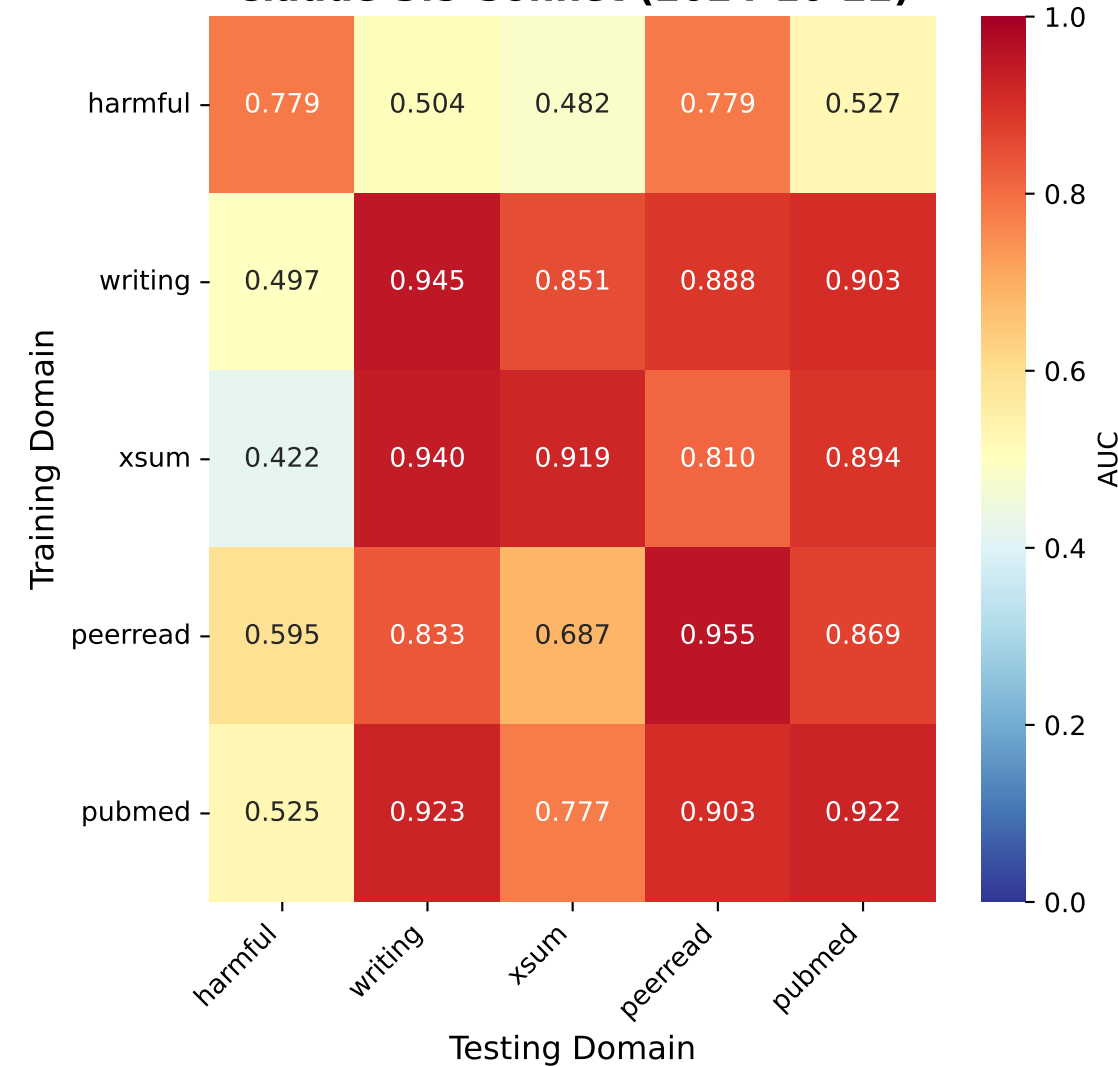
Claude-3.5-Sonnet (2024-10-22)
