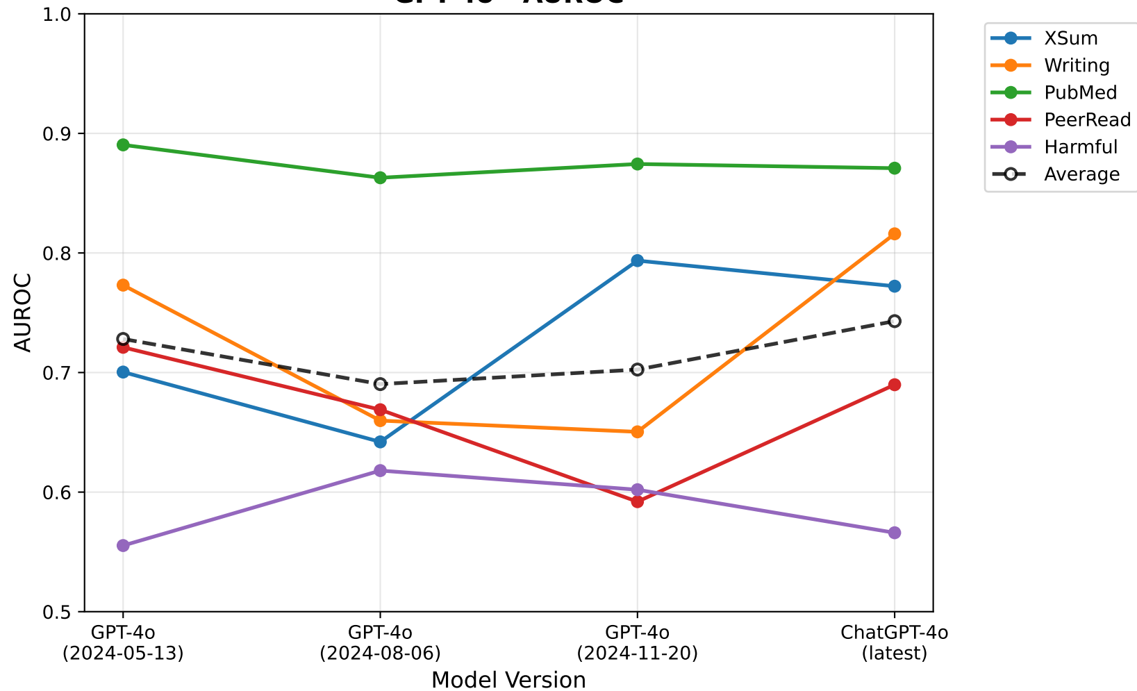
GPT-4o - AUROC
