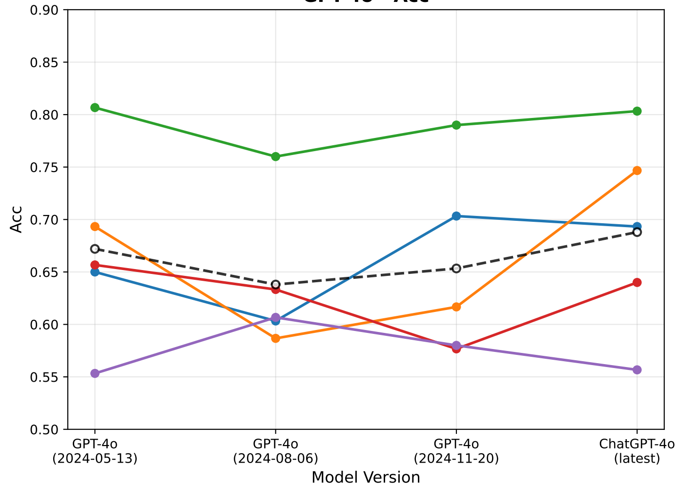
GPT-4o - Acc
