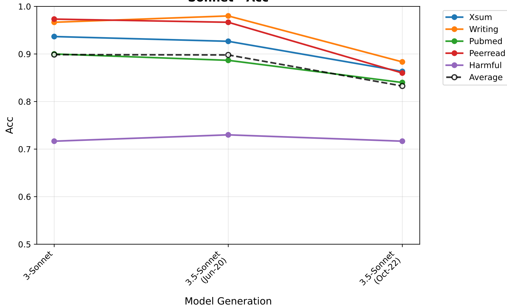
Sonnet - Acc
