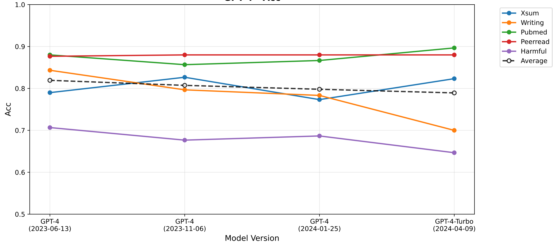
GPT-4 - Acc
