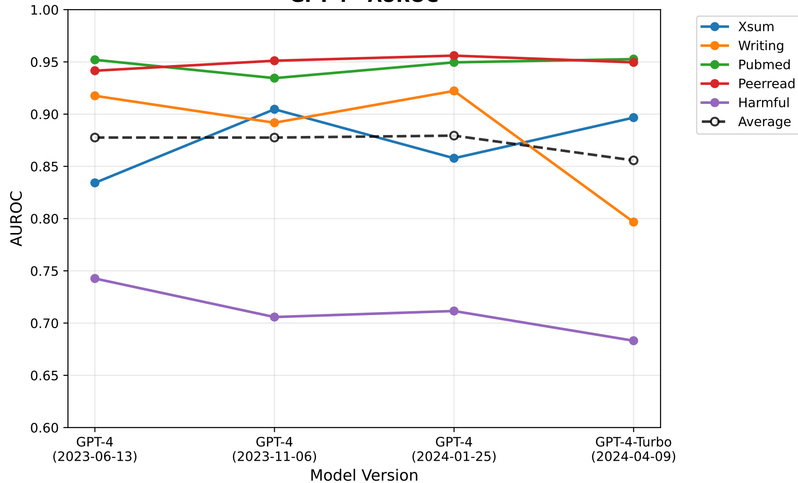
GPT-4 - AUROC
