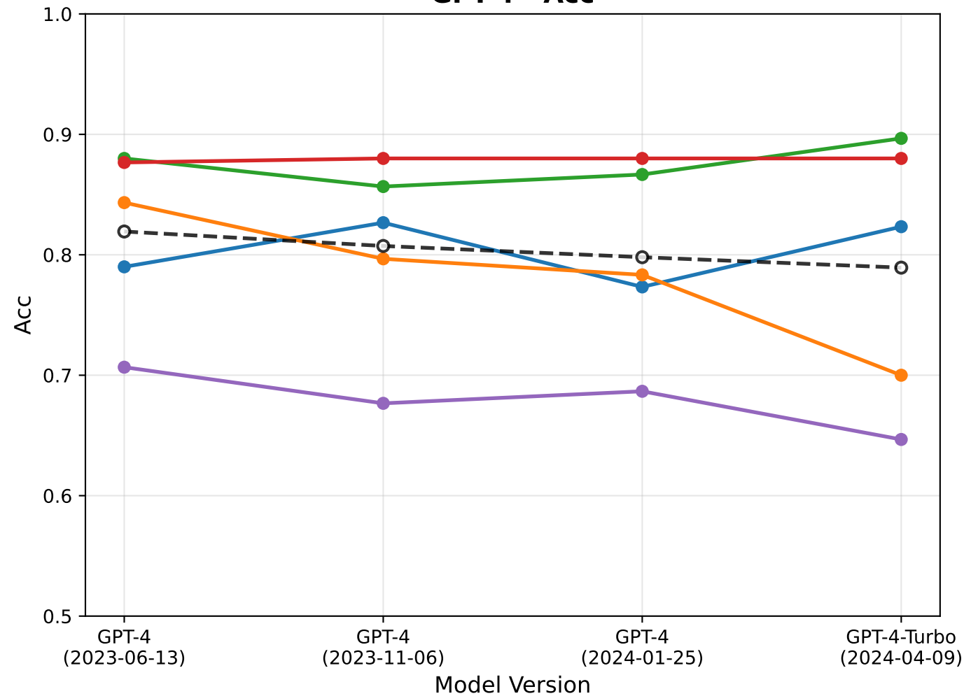
GPT-4 - Acc
