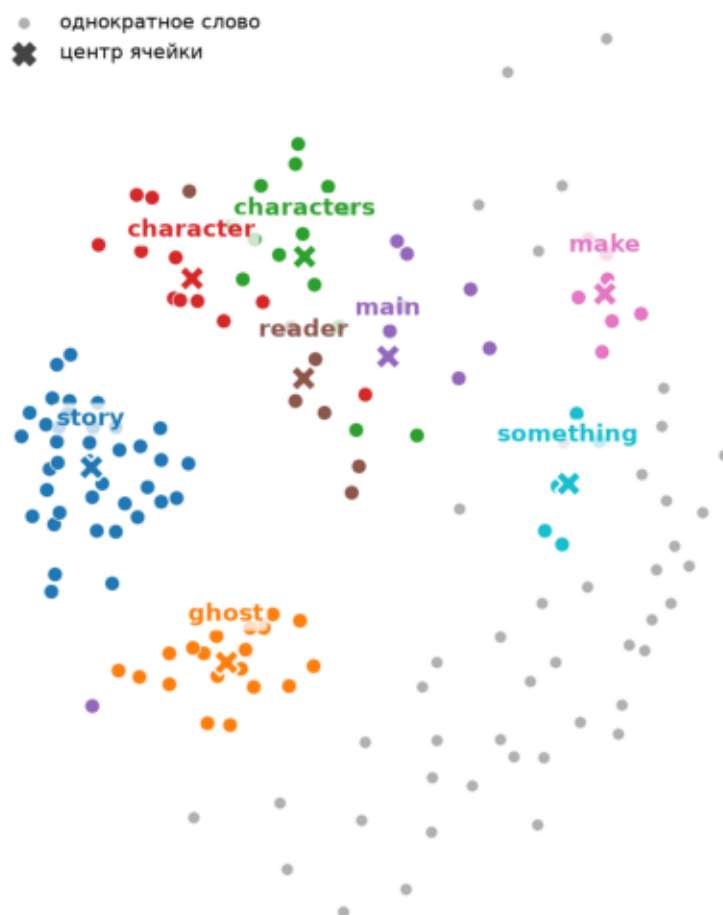
Ячейки смысловых слов, текст 50: каждый тип своим цветом, центр — крестом
