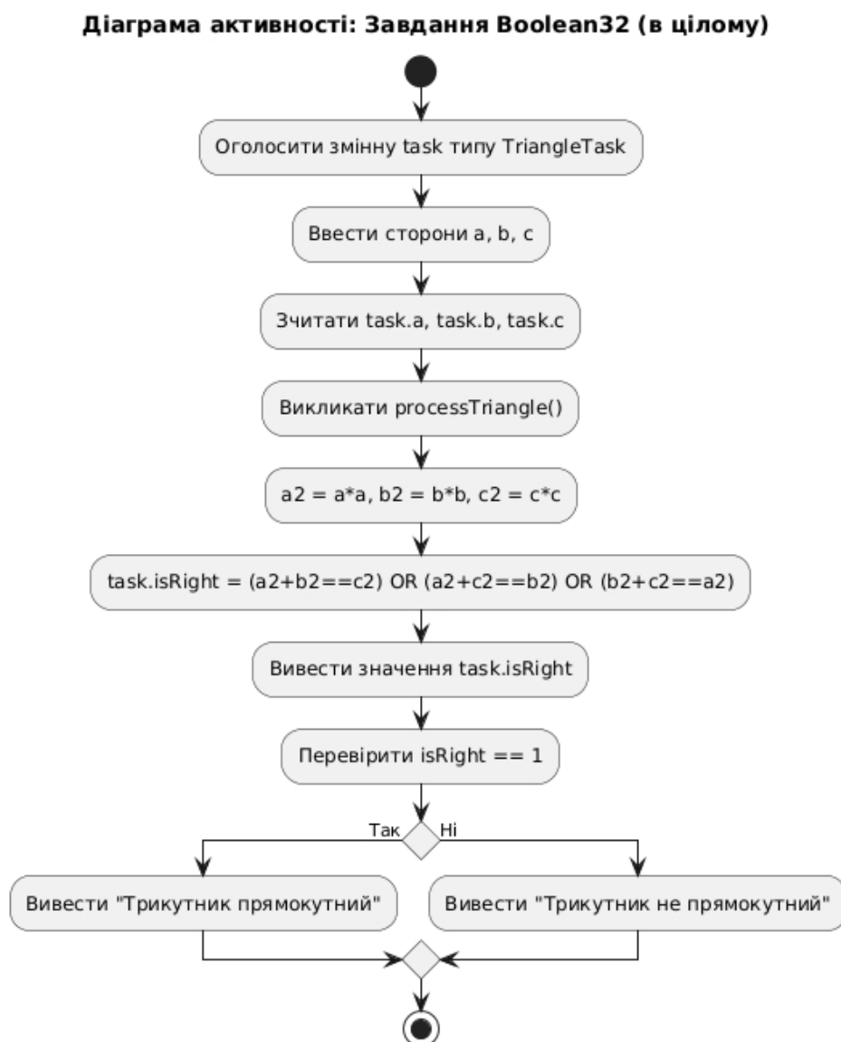
Рисунок 1.3 – Діаграма активності до задачі Boolean32.
