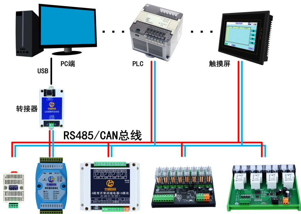
图 1.1 电源与通讯接线示意图 1.4.3 RS485 总线通讯接线
