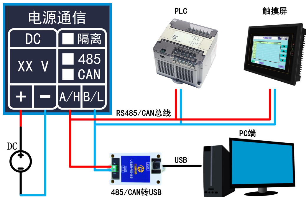
图 1.1 电源与通讯接线示意图 1.4.3 RS485 总线通讯接线
