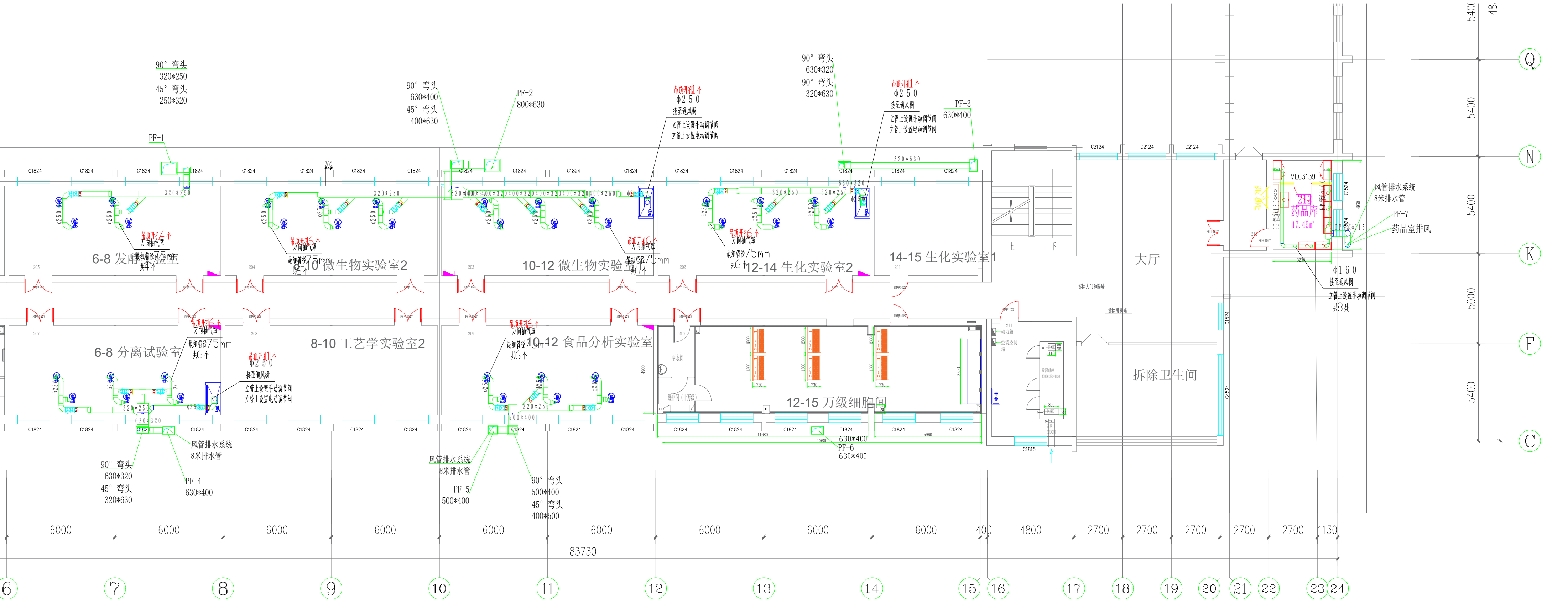
二层通风平面图 1:150
