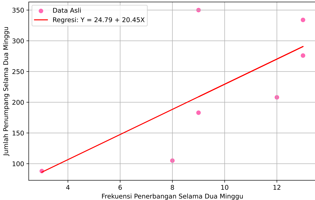
Regresi Linier Frekuensi vs Jumlah Penumpang
