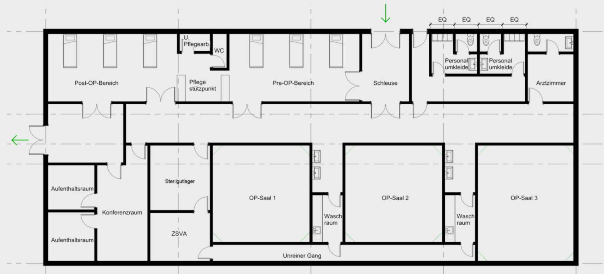
GRUNDRISS - OG | OP - BEREICH
