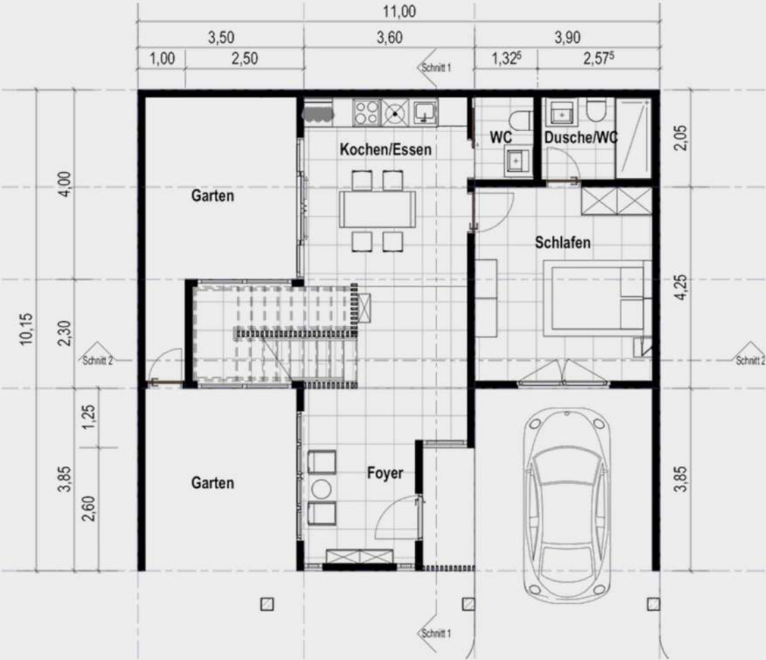
GRUNDRISS - EG
