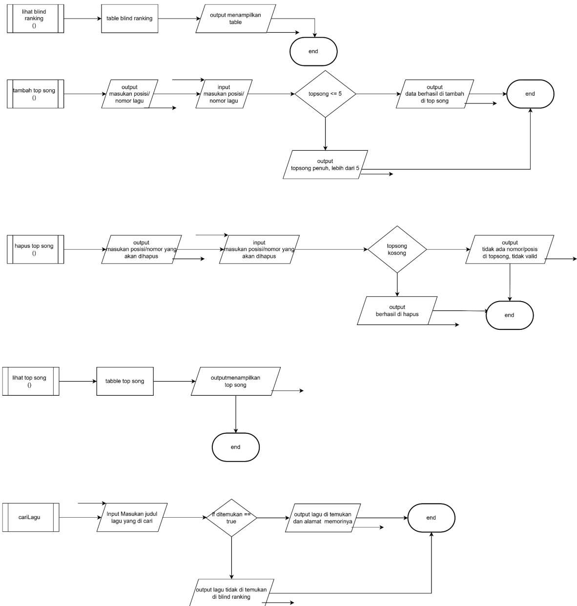
Gambar 1.7 (Fungsi lihat blind ranking, tambah top song, hapus top song, lihat top song, carilagu, dan keluar)
