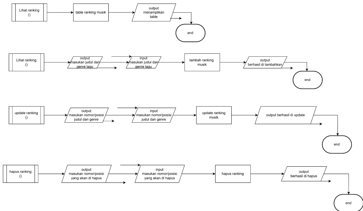
Gambar Flowchart 1.5 (Fungsi lihat, tambah, update, hapus, keluar)
