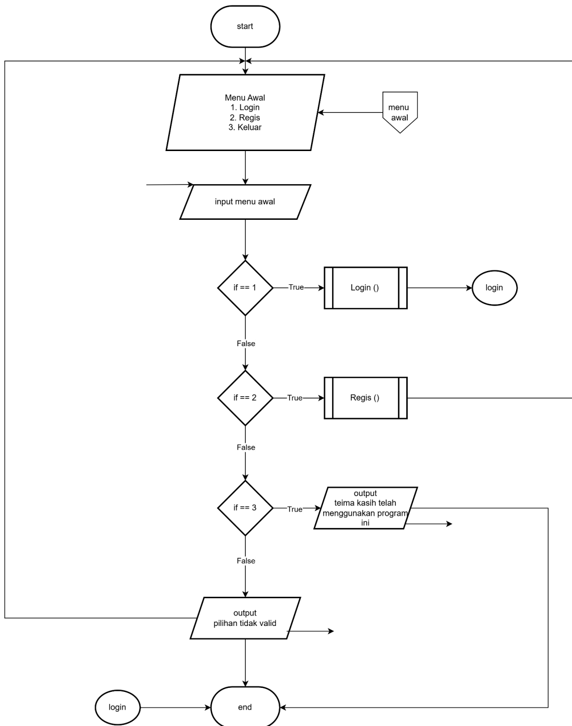
Gambar Flowchart 1.1 (menu awal, (regis), (login), (keluar))
