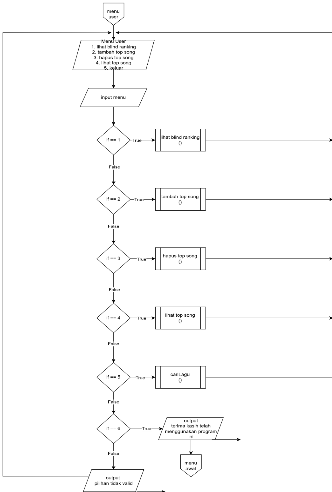
Gambar Flowchart 1.6 (Menu User, bagian user)
