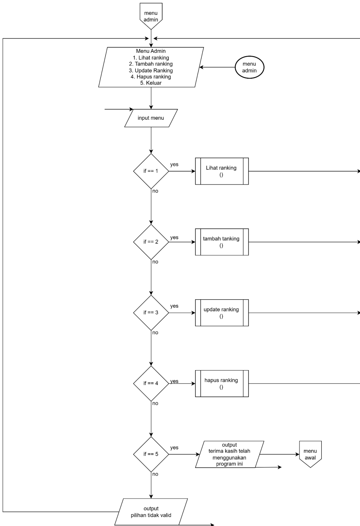
Gambar Flowchart 1.3 (menu admin, bagian admin)
