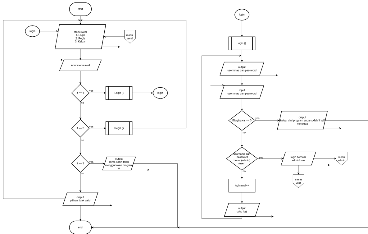
Gambar Flowchart 1.1 (menu awal, (regis), (login), (keluar) dan fungsi login)
