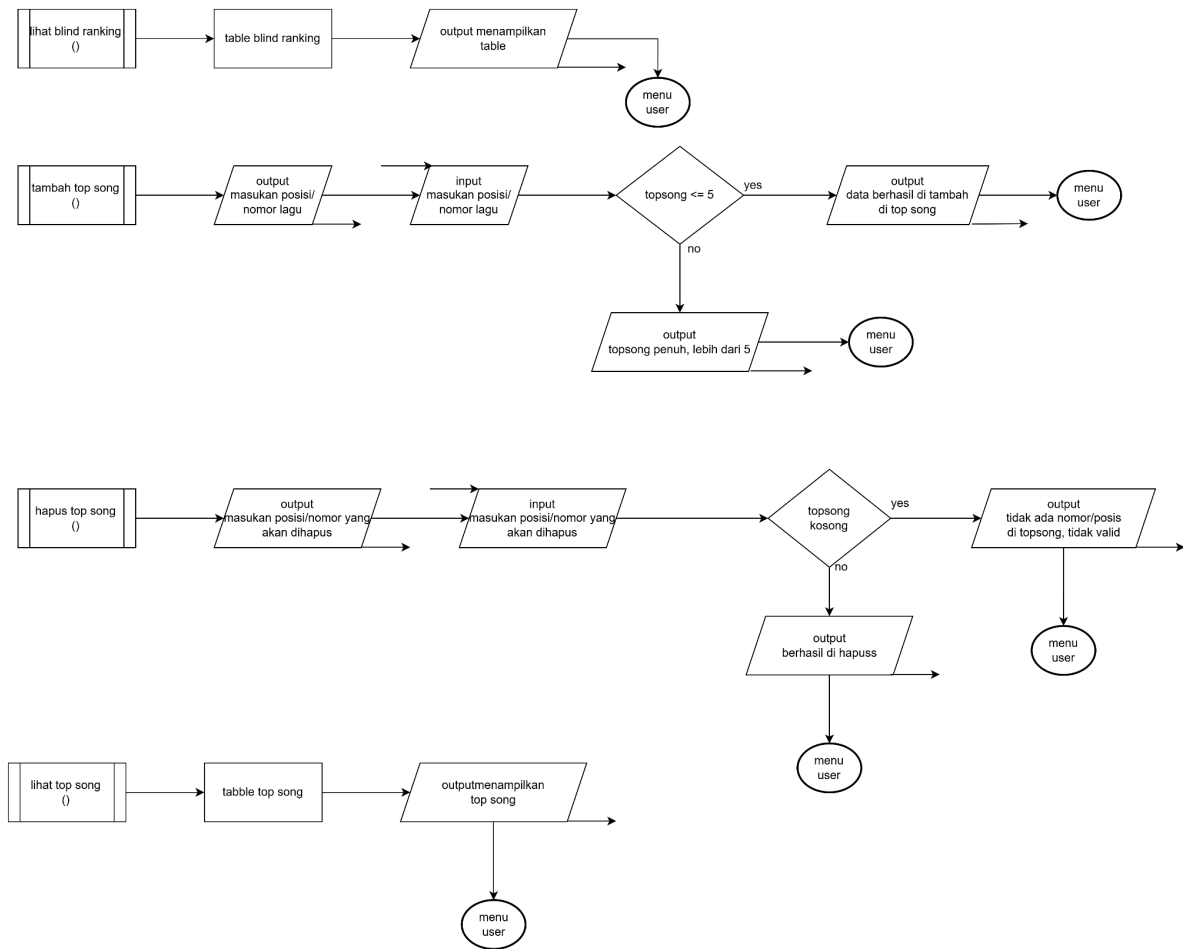
Gambar 1.6 (Fungsi, lihat blind ranking, tambah top song, hapus top song, lihat top song, keluar)
