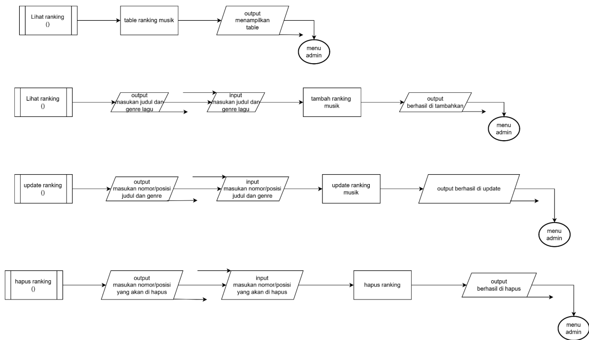
Gambar Flowchart 1.4 (Fungsi lihat, tambah, update, hapus, keluar)
