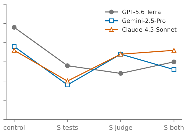
LiveCodeBench
