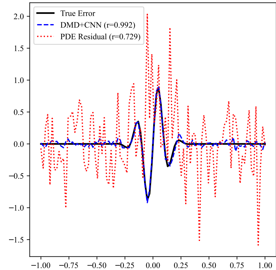
a. 1D Allen-Cahn Error Dynamics
