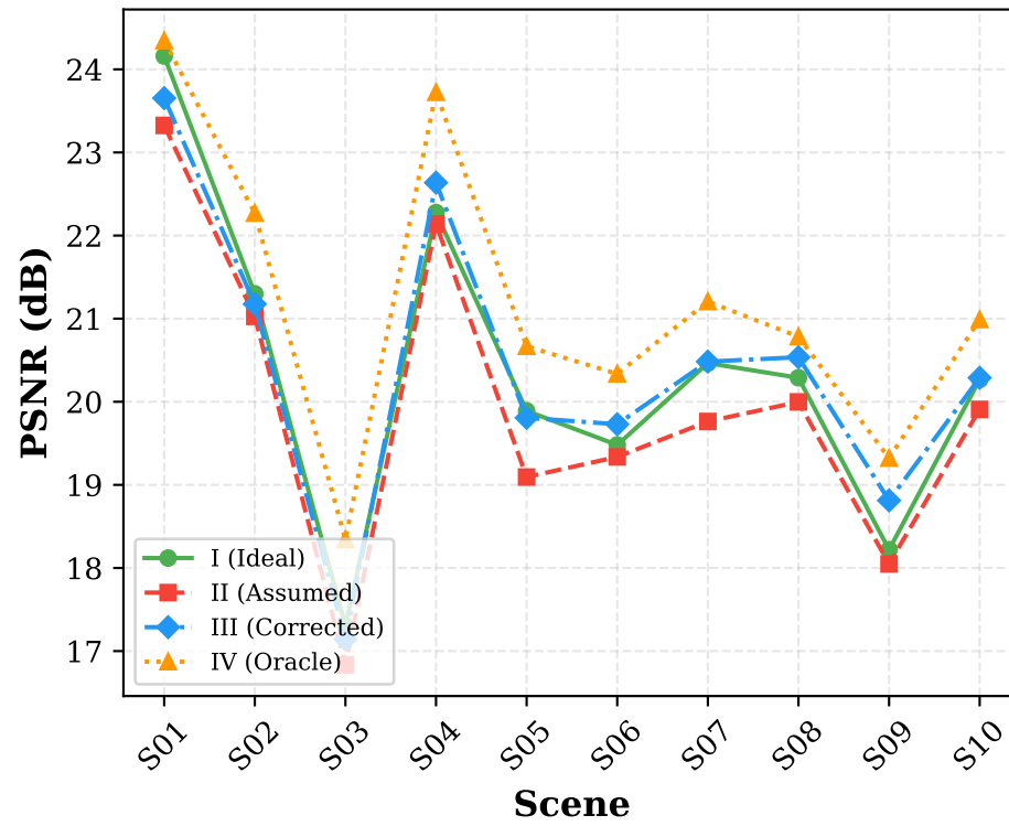
HDNet
