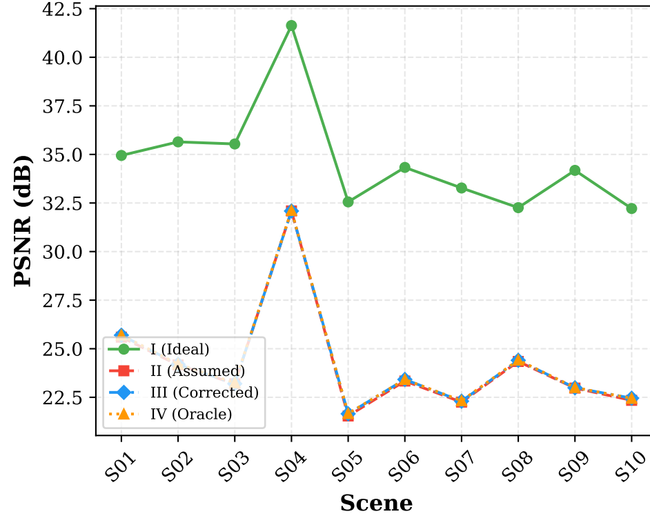
HDNet
