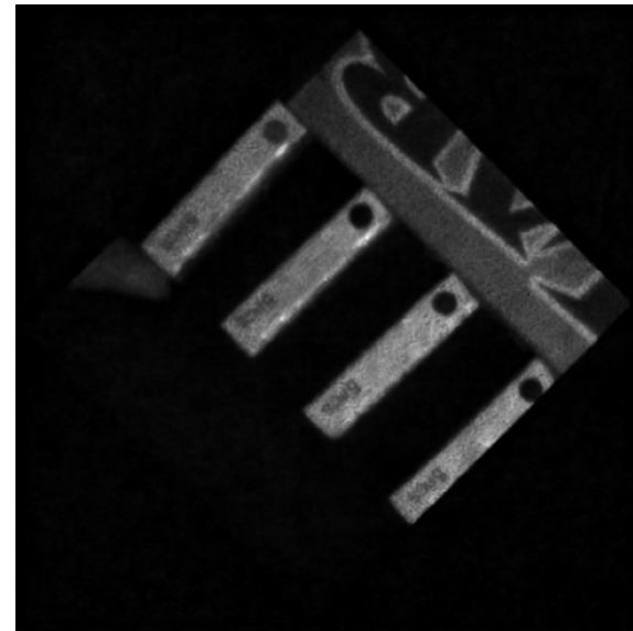
EfficientSCI (Mis.)
