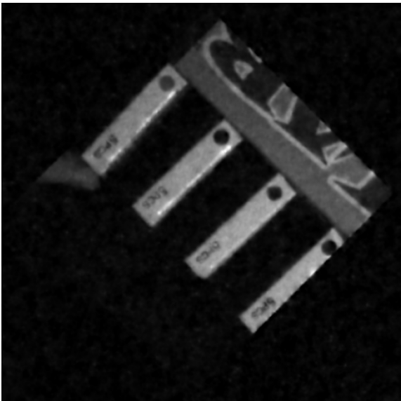
GAP-TV (Cal.)
