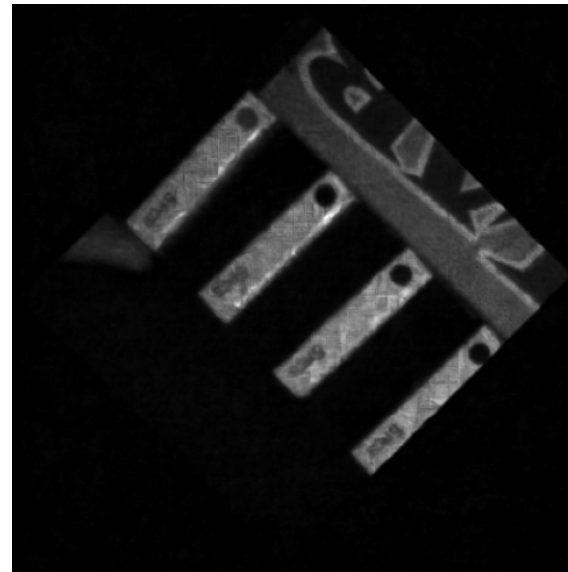
EfficientSCI (Cal.)
