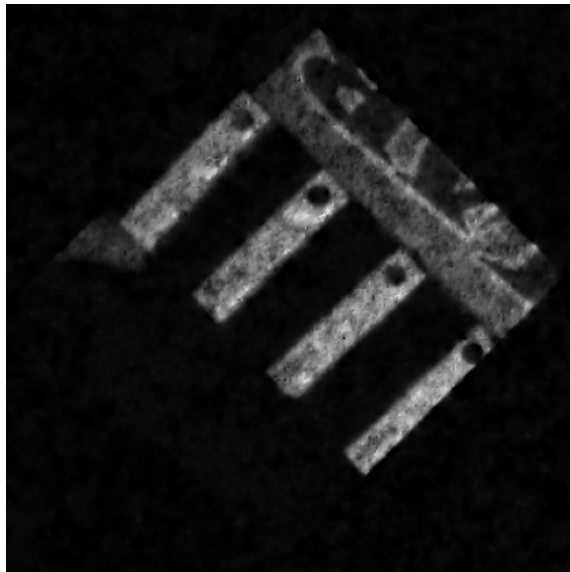
GAP-TV (Mis.)
