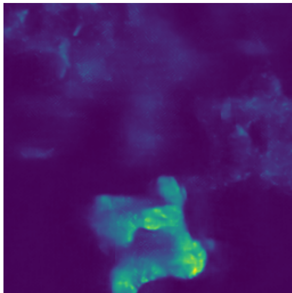
HDNet
