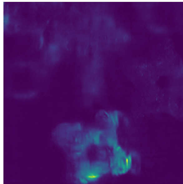
MST-S
