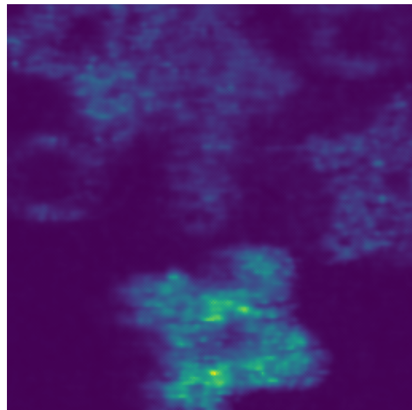
GAP-TV
