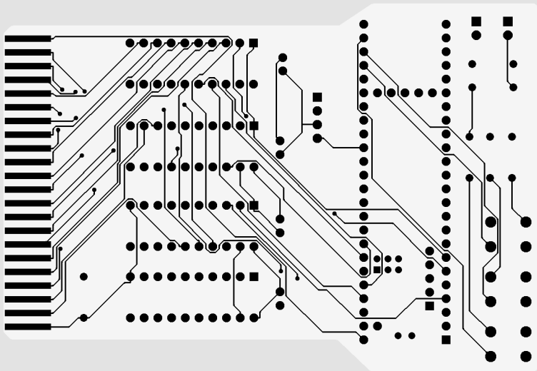
E1819670 BOTTOM layer Image (topview)
