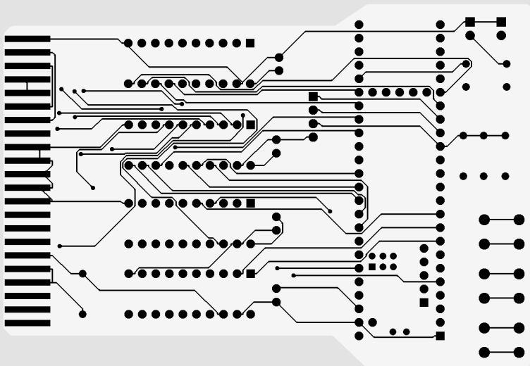
E1819670 TOP layer Image (topview)
