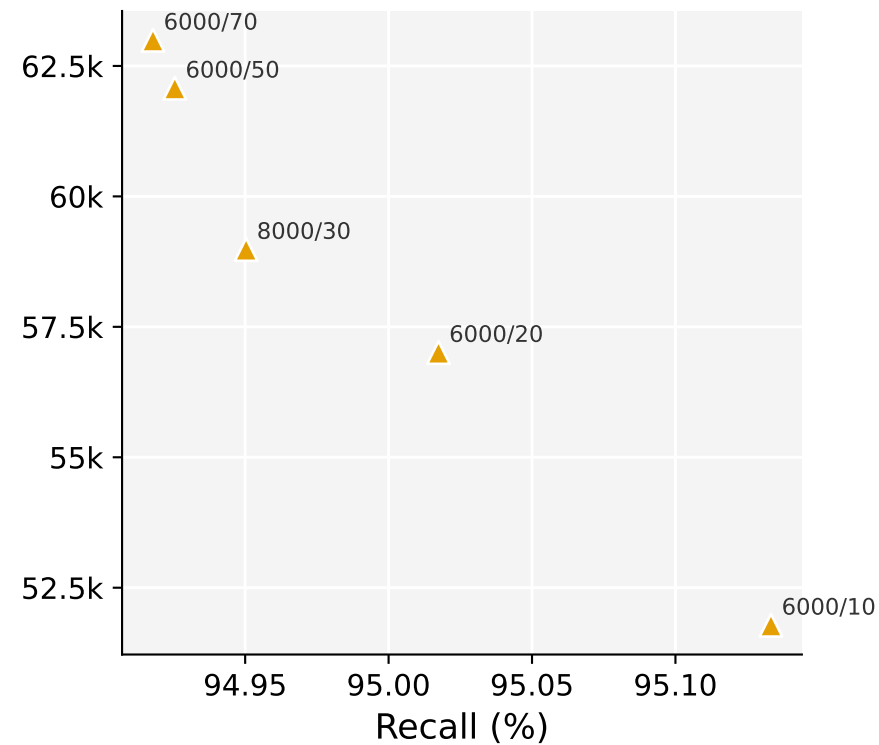
FreshDiskANN-BriskSeed
