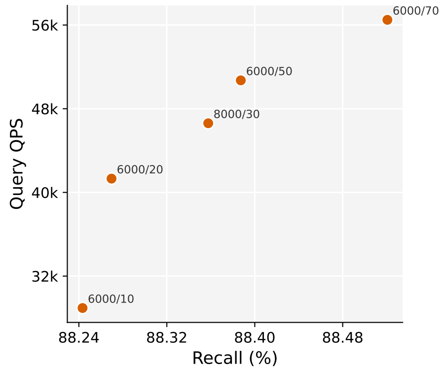
HNSW-BriskSeed
