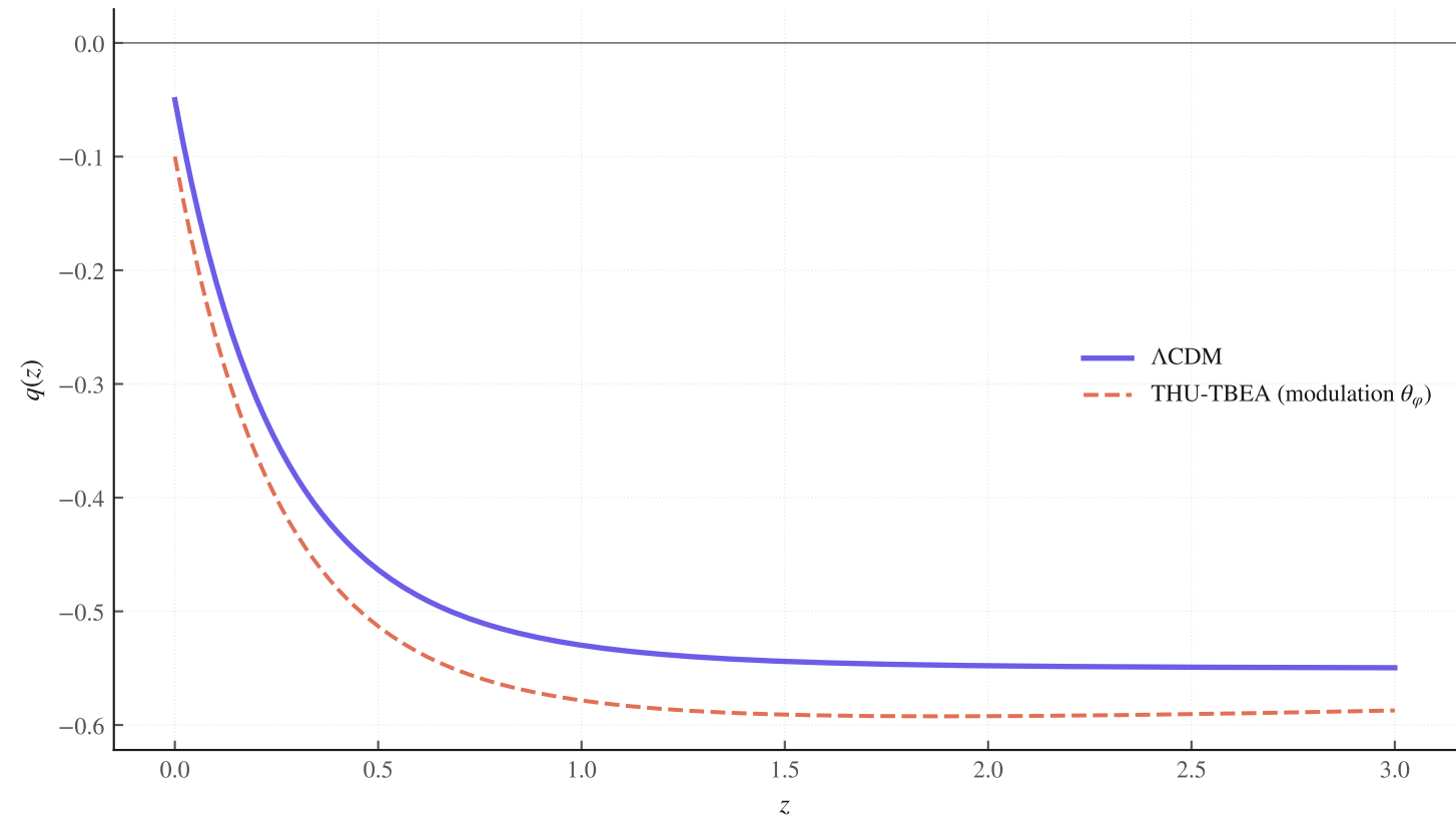
Deceleration parameter q(z) - prediction P1
