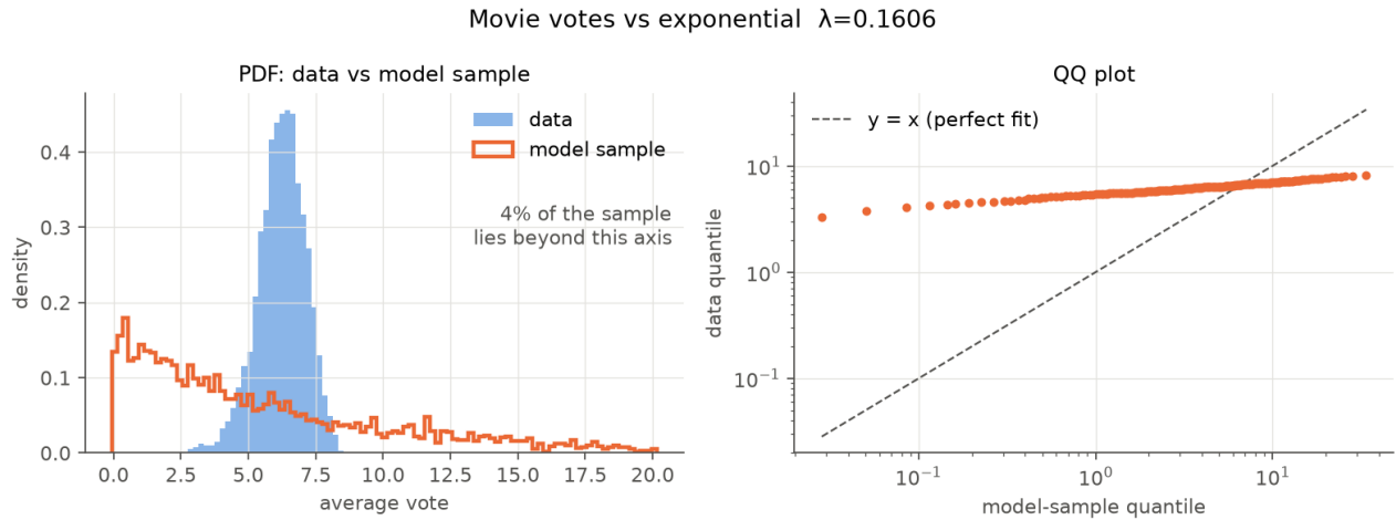
Figure 9: 영화 평점에 지수분포 ( \hat{\lambda} = 0.1606 ) 를 적합한 결과 (code/p1.py 가 생성). D = 0.490 .
