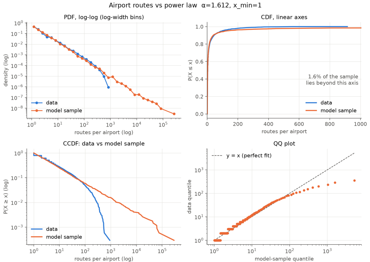
Figure 7: 공항 노선 수에 멱법칙 ( \hat{\alpha} = 1.612 , x_{\min} = 1 ) 을 적합한 결과 (code/p1.py 가 생성). D = 0.209 .
