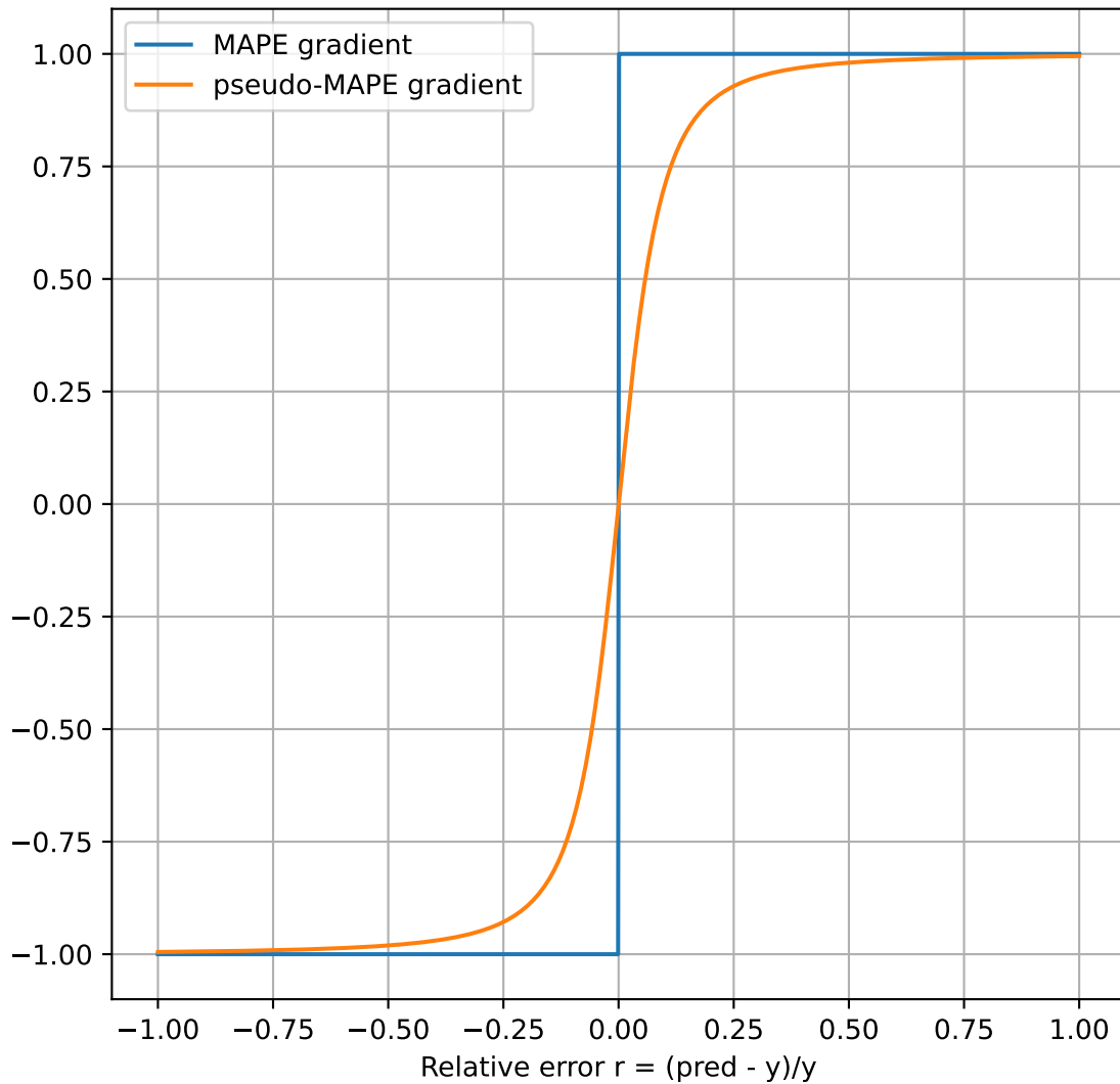
Gradients
