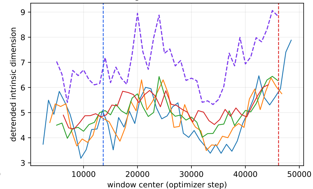
gradient norm
