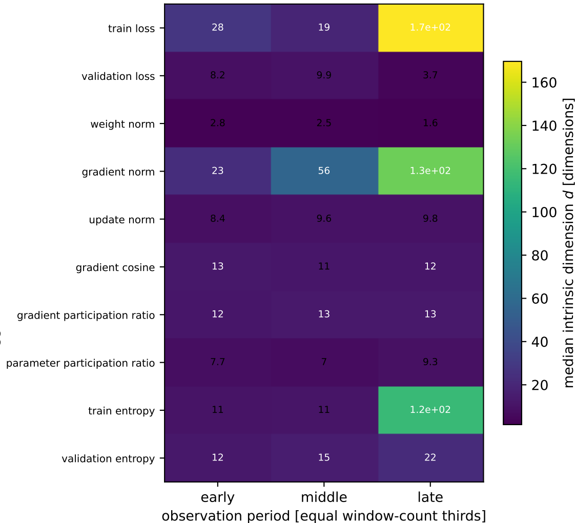
LB median (linear colour scale)
