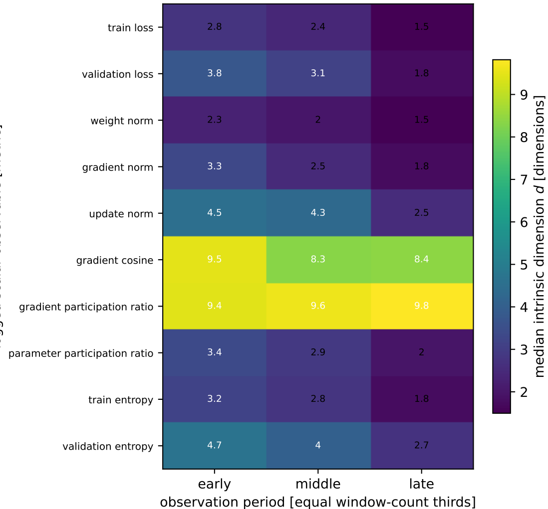
MG median (linear colour scale)
