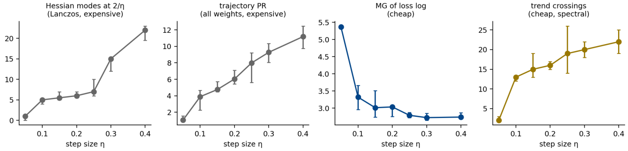
Рис. 2: Уровни по шагу \eta : два дорогих эталона растут, MG падает.
