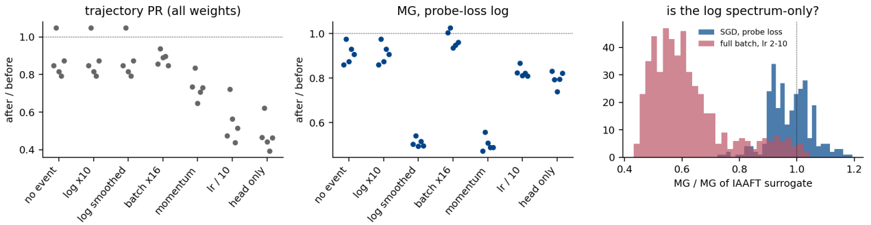
Рис. 1: Пилот. Слева и в центре — отношение после/до для эталона и для MG лог loss на фиксированном probe. Справа — распределение MG/MG суррогата по окнам: под SGD оно сосредоточено у 1, в полнобатчевом режиме с большим шагом — заметно ниже 1.
