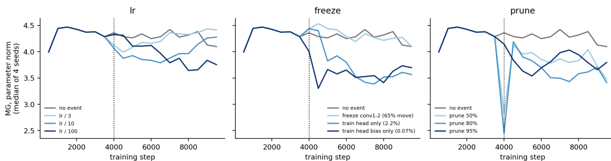
Рис. 6: MG во времени, медиана по 4 седам. При прунинге окно, накрывающее сам шаг 4 000, падает до \approx 2.4 : норма там скачком меняется. Такие окна в сравнение не входят — «после» начинается с шага 5 000.
