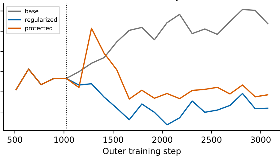
MG, W=512, delay=1
