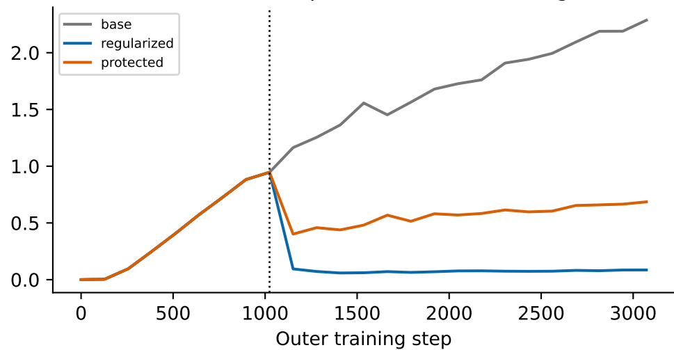
MG, W=512, delay=1
