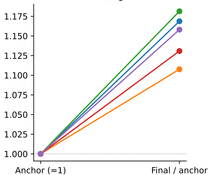
Scalar MG, right knee
