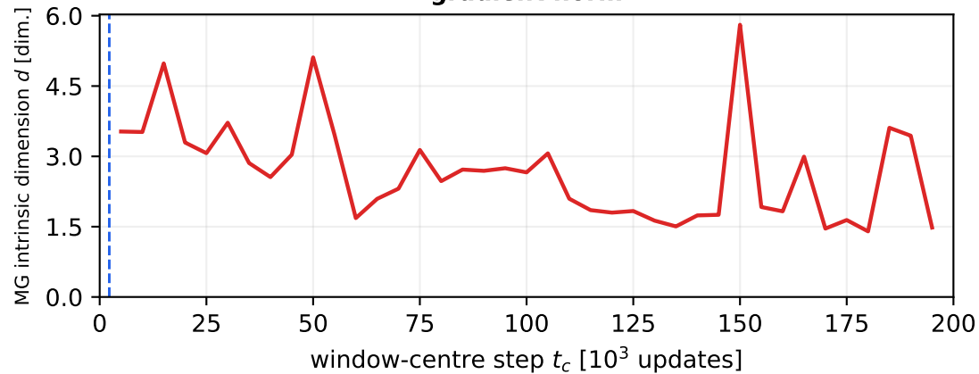
gradient norm
