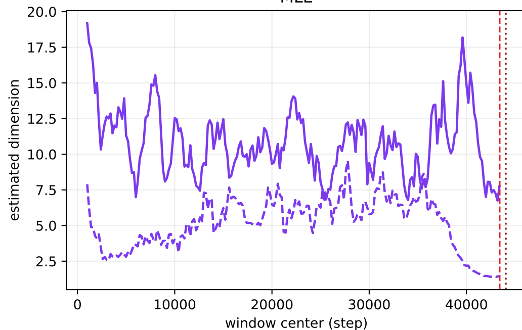
MLE
